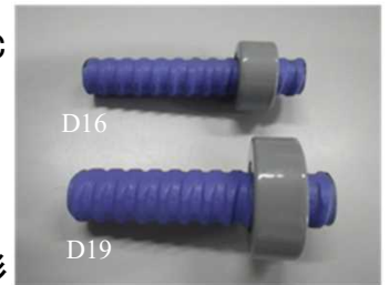
円形ナット:FCD450-10 エポキシ樹脂塗装:高付着型
